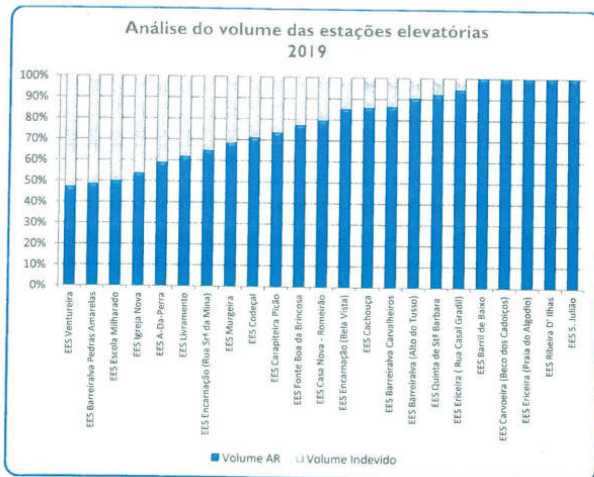
Gráfico 13 – Volumes das Estações Elevatórias
